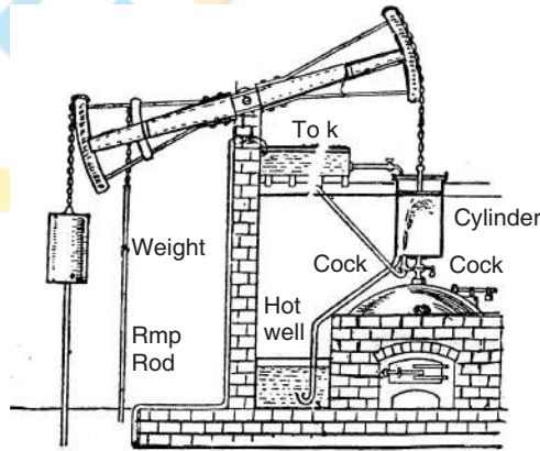
चित्र 5 न्यू कॉमन का इंजन
